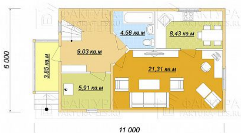
План первого этажа
