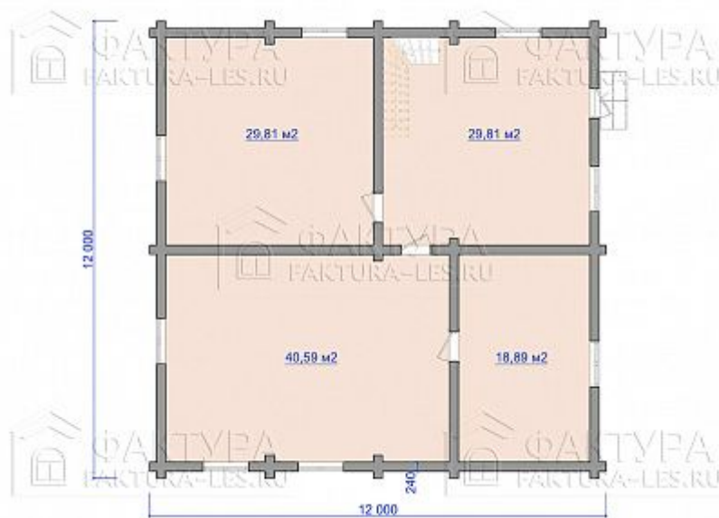
План 1 этажа
