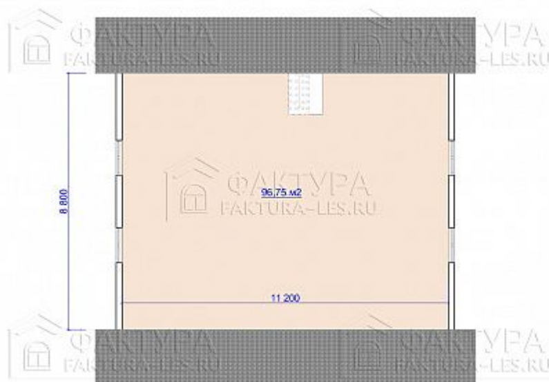
План 2 этажа
