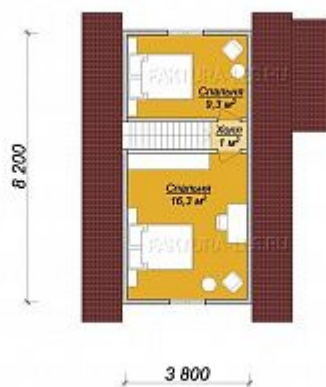
План второго этажа
